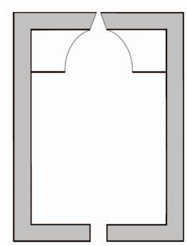
Şəkil-plan 10. Kərimli alban məbədinin planı (T.V.Əliyev)
